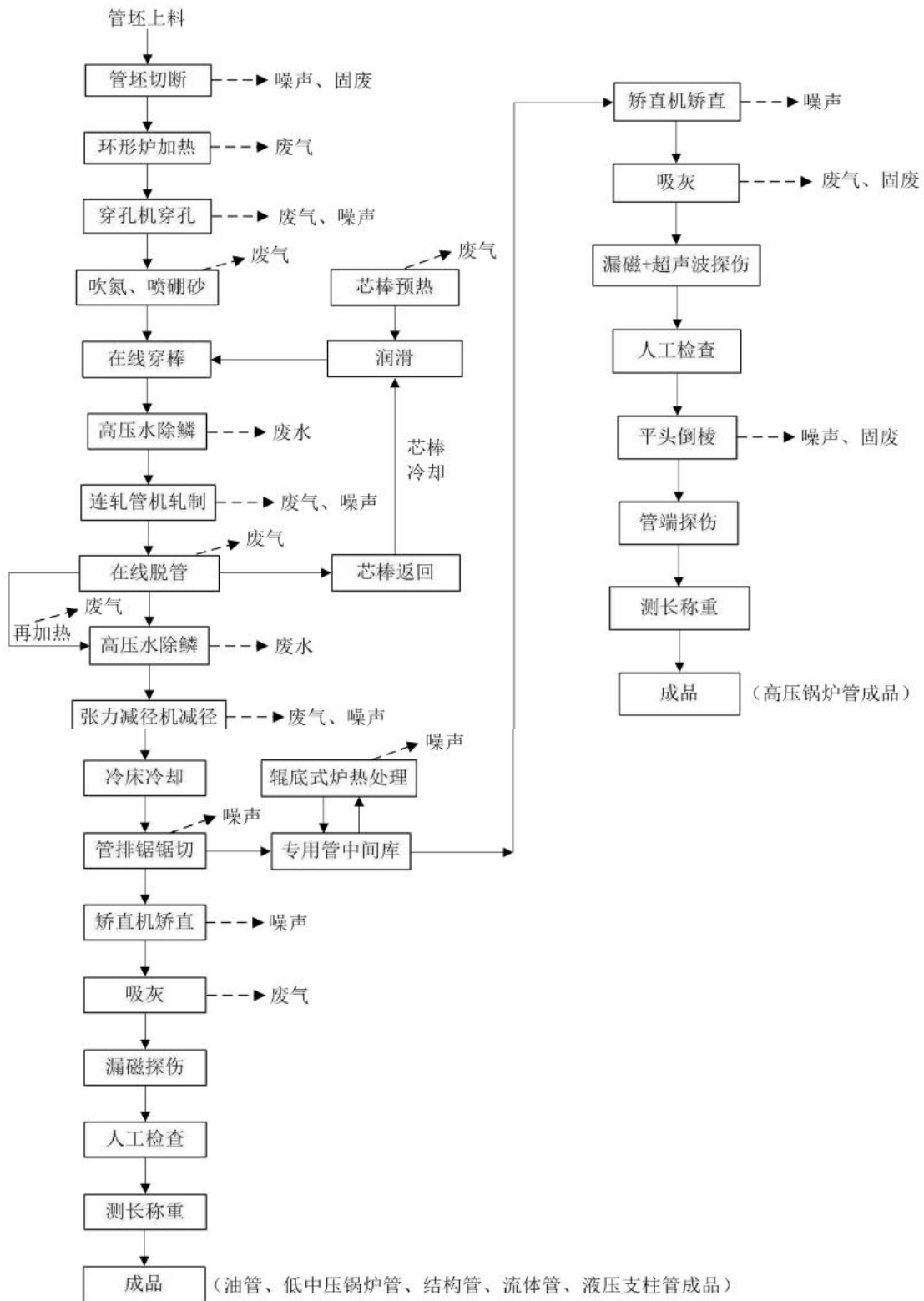
图 4.5-22 特种钢管生产工艺流程图
