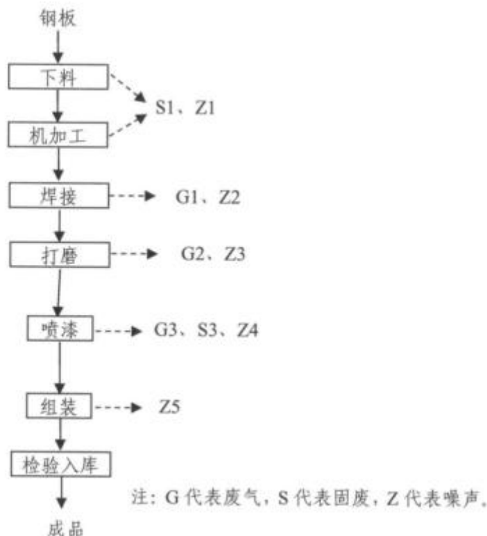
图 4.4-3 升降机械工艺流程
