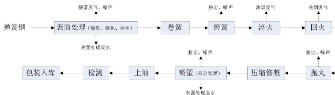
图 4.5-23 弹簧生产工艺流程图
