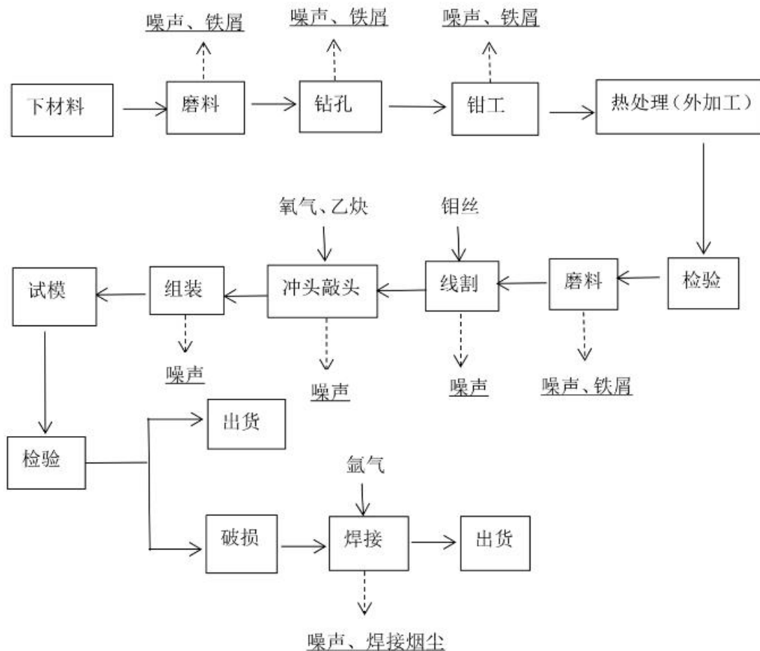
图 4.5-17 五金制品生产工艺流程图
