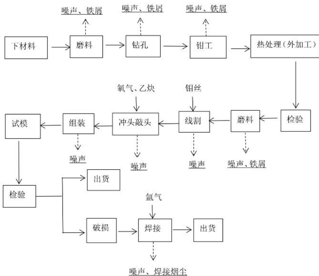
图 4.5-12 模具生产工艺流程
