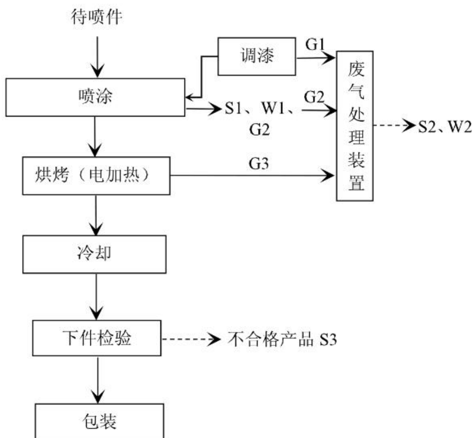
图 4.5-11 苏州锦毅昌电子有限公司汽车、配件工艺流程
