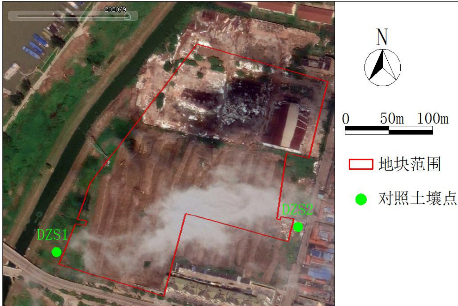
图 4.1.3-5 洪新河安置房地块-4 对照点位布置图 (以 2020 年 9 月历史影像为底图)
