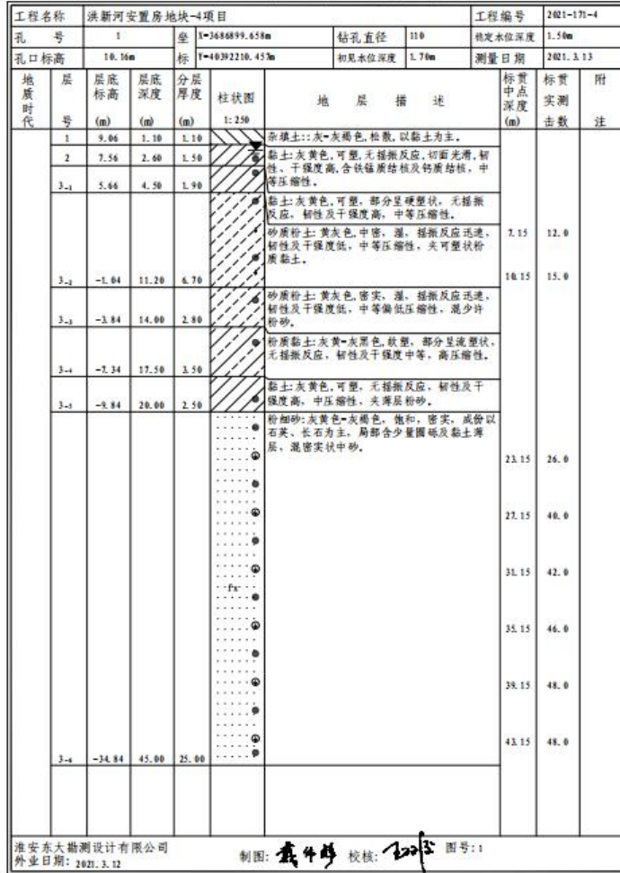
钻孔柱状图
