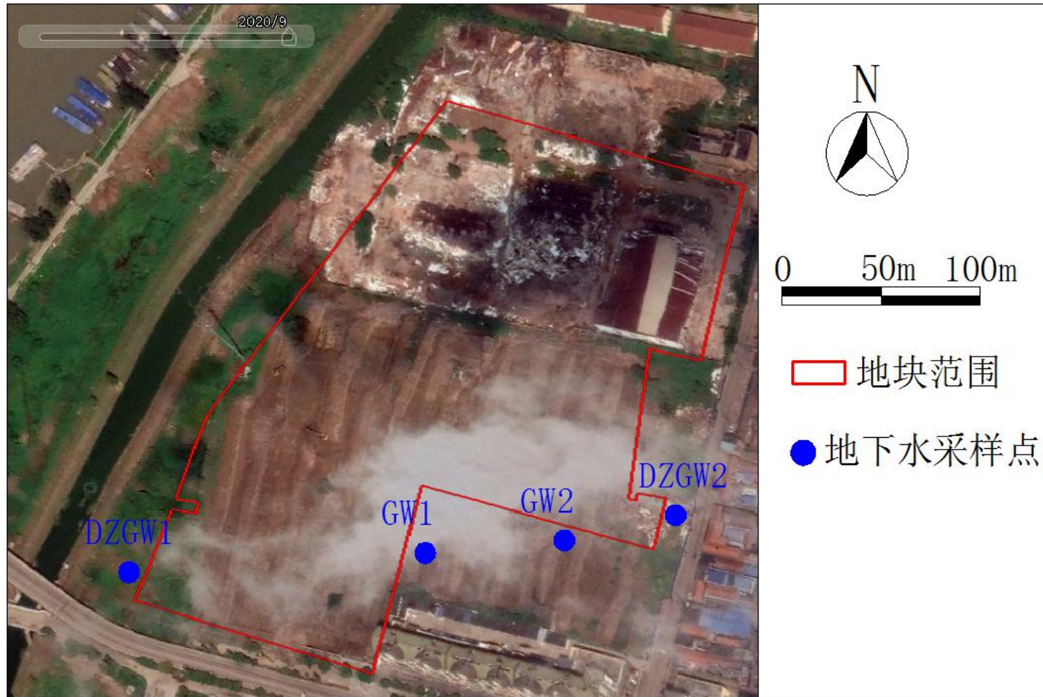
图 4.1.3-6 洪新河安置房地块-4 周边地下水点位布置图（以 2020 年 9 月历史影像为底图）
