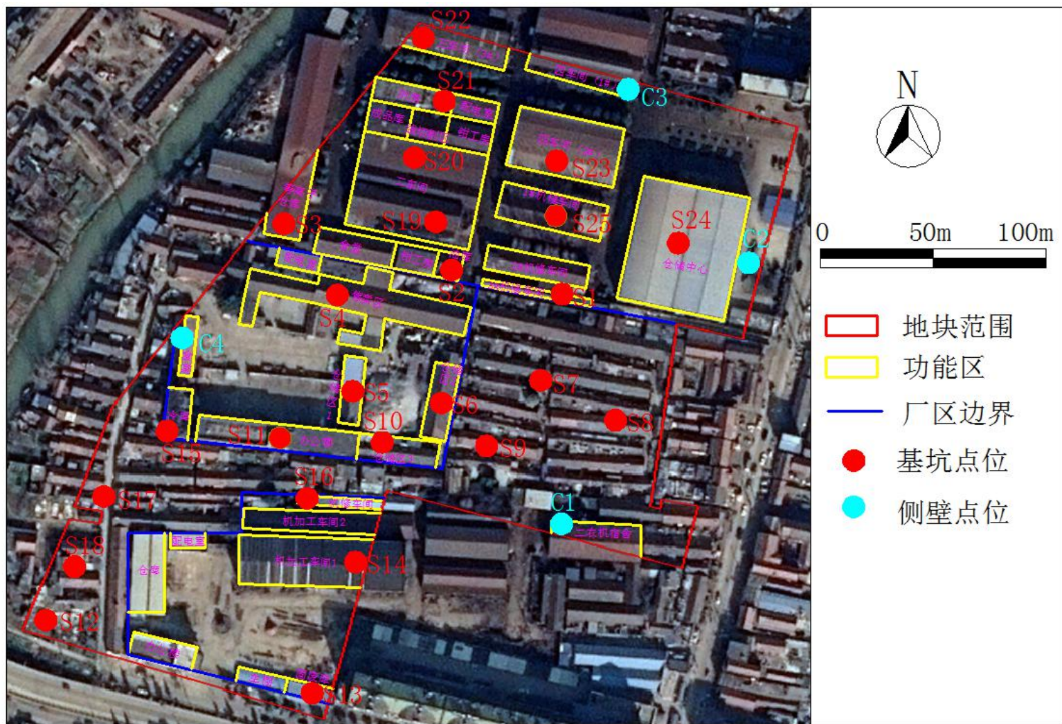
图 4.1.3-1 洪新河安置房地块-4 地块点位布置图（以 2013 年 12 月历史影像为底图）
